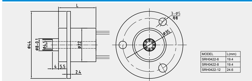
标准型 Standard Type SRH0422
